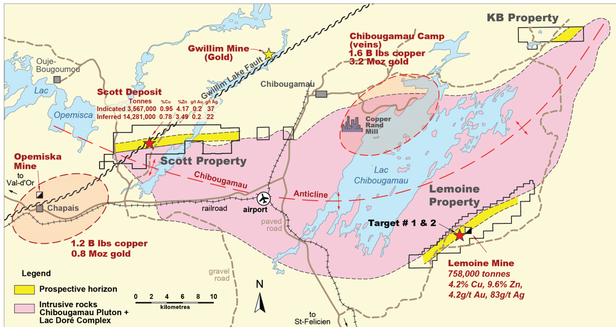
Figure 1. Carte de localisation des projets de Yorbeau dans le camp minier de Chibougamau, Québec, incluant la propriété Lemoine.
